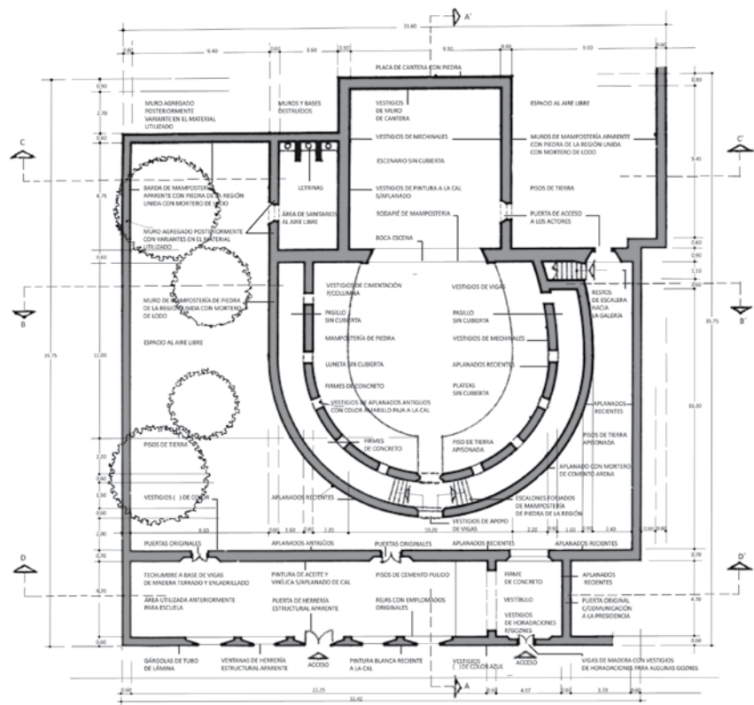
Planta Baja. Levantamiento de materiales, daños y deterioros
