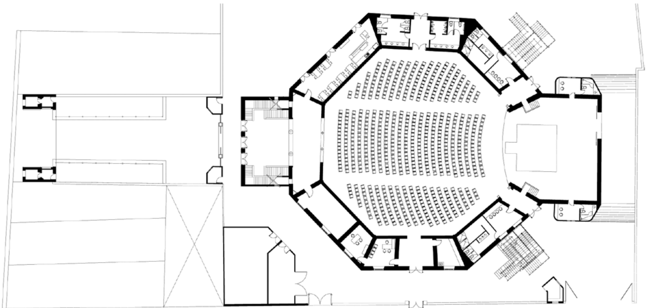
Planta baja
