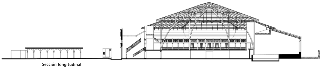
Sección longitudinal
