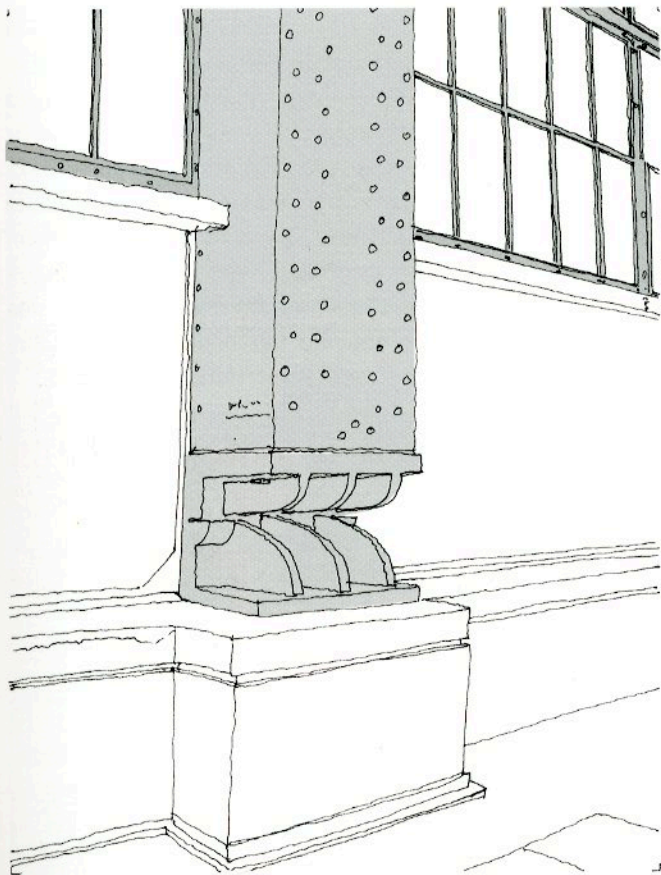
Detalle de la estructura, Fábrica de turbinas AEG
