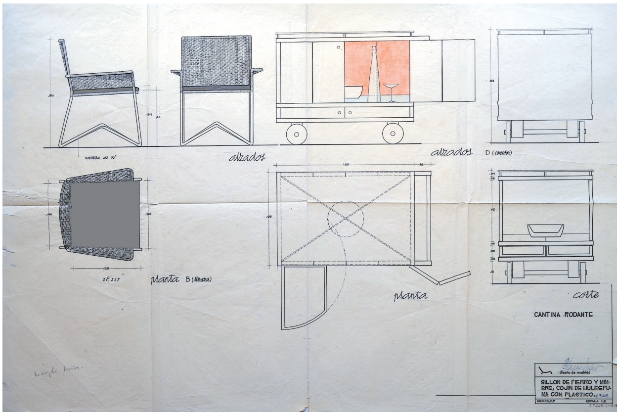
Sillón de fierro y mimbre, cojín de hule espuma con plástico y cantina rodante, entrada CP 328-1-10-10 del Archivo
