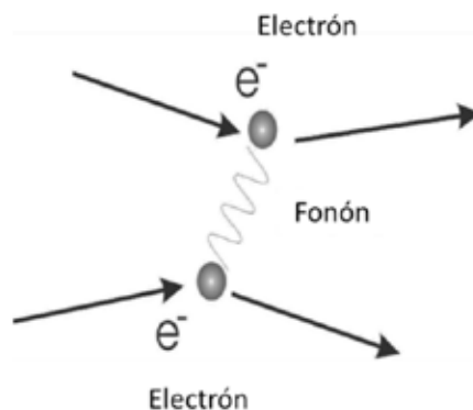
Figura 2 Interacción electrón-fonón-electrón
