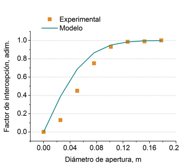
Figura 3. Influencia del diámetro de apertura sobre el factor de intercepción
