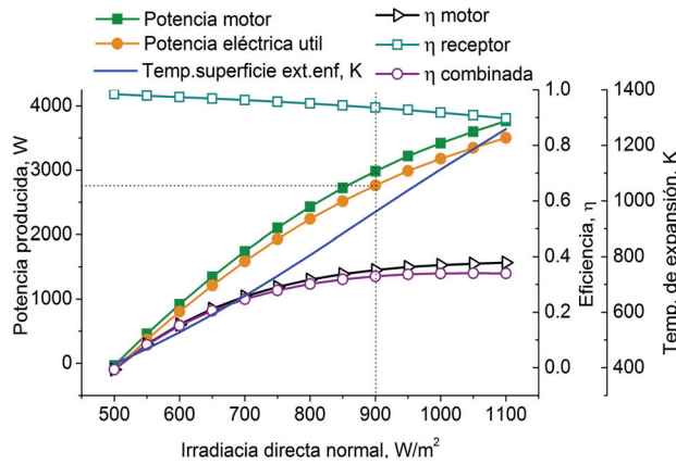
Figura 10. Influencia de la irradiancia solar directa sobre la potencia
