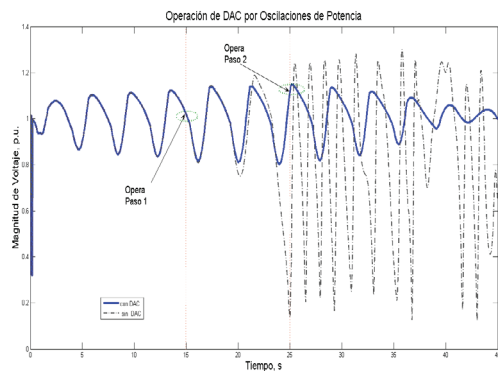
Figura 14. Identificación de frecuencias críticas modo de oscilación interárea Norte-Sur
