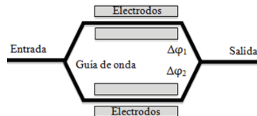
Figura 1. Modulador MZ de control doble
