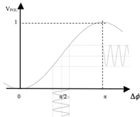
Figura 2. Curva de transferencia de potencia de un modulador MZ
