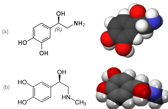
Figura 1. Noradrenalina y adrenalina (fórmulas químicas y “de bolas”): (a) Noradrenalina, (b) Adrenalina.
