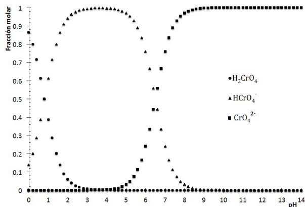
Figura 1. Diagrama de distribución de especies del ácido crómico en función del pH. Las constantes de disociación ácida utilizadas para el \text{H}_2\text{CrO}_4 son: K_{a1} = 10^{-0.8} y K_{a2} = 10^{-6.5} (Burriel, 1989).
