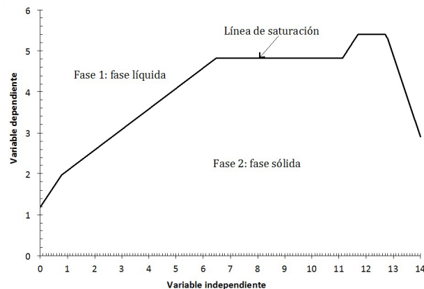
Figura 2. Representación general de un diagrama de existencia-predominio.
