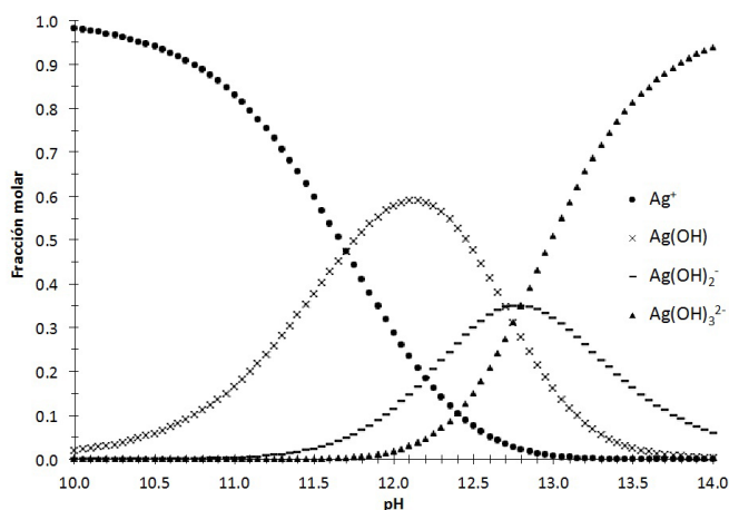
Figura 4. Diagrama de distribución de especies para el sistema \text{Ag}^+ - \text{H}_2\text{O} en función del pH. Las constantes utilizadas son las mostradas en la escala de pH, K_{a1} = 10^{-1.17} , K_{a2} = 10^{-12.7} y K_{a3} = 10^{-12.8} (Ringbom, 1979).
