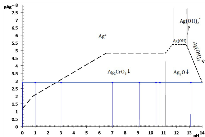
Figura 5. Diagrama de existencia predominio para el sistema \text{Ag}^+ - \text{CrO}_4^{2-} - \text{H}_2\text{O} , válido a 5.0 \times 10^{-3} M de cromato. Se muestran los valores de pH experimentales. El doble apóstrofe en \text{pAg}'' denota la dependencia del pH y \text{pCrO}_4' .
