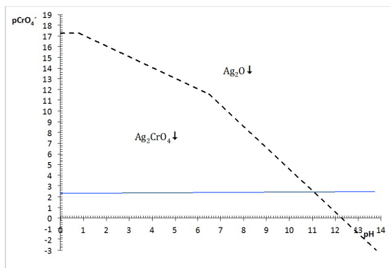
Figura 3. Diagrama de fases condensadas para el sistema \text{CrO}_4^{2-} - \text{Ag}^+ - \text{H}_2\text{O} en el plano \text{pCrO}_4'/\text{pH} .
