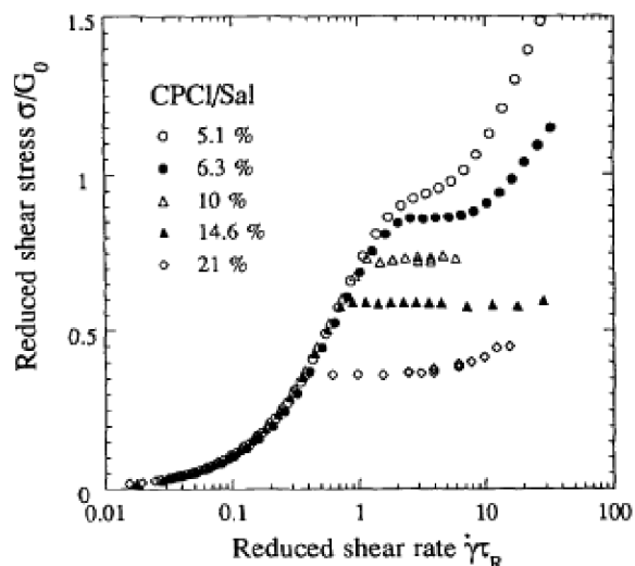
Figura 6. Curva de flujo de esfuerzo reducido en función de la velocidad de corte reducida, para varias concentraciones del surfactante. Solución micelar de cloruro de cetilpiridinio con salicilato de sodio (Berret et al. , 1997).
