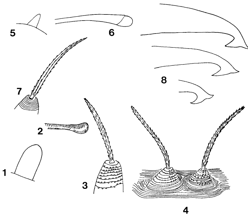
Figs. 1-8. 1-4. Hembra de Mononychellus hoffmannae sp. nov. 1, eupatidio (sensilo terminal) del tarso-palpo, su \zeta ; 2, peritrema: porción distal; 3, sedas dorso-opistosomales, c2 ; 4, Estriación dorso-opistosomal central y alrededor de tubérculos sedales. 5-8: Macho de Mononychellus hoffmannae sp. nov. 5, eupatidio (sensilo terminal) del tarso-palpo, su \zeta ; 6, peritrema: porción distal; 7, sedas dorso-opistosomales; 8, aedeagus, mostrando variaciones.
